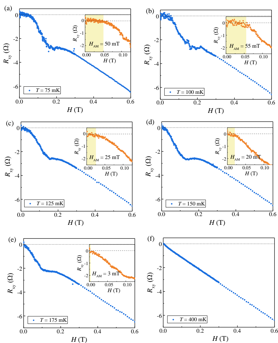
图 S1 不同温度下的霍尔电阻 R_{xy}
