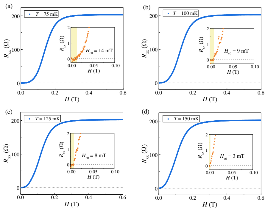
图 S2 不同温度下的纵向电阻 R_{xx}
