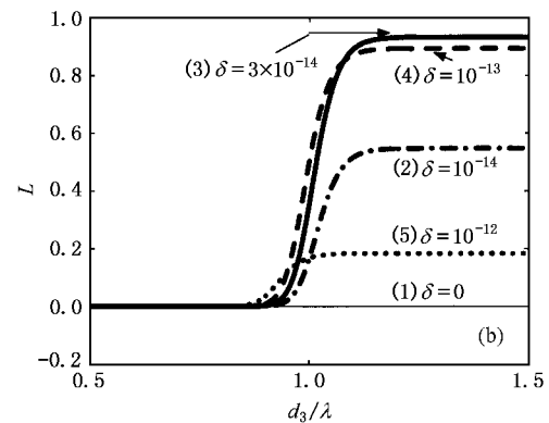
图 3 在不同损耗参数下 (a) 能量透射率 (b) 能量损耗率随平板厚度 d_3 的变化,这时 k_x = 2\sqrt{2}k_0
