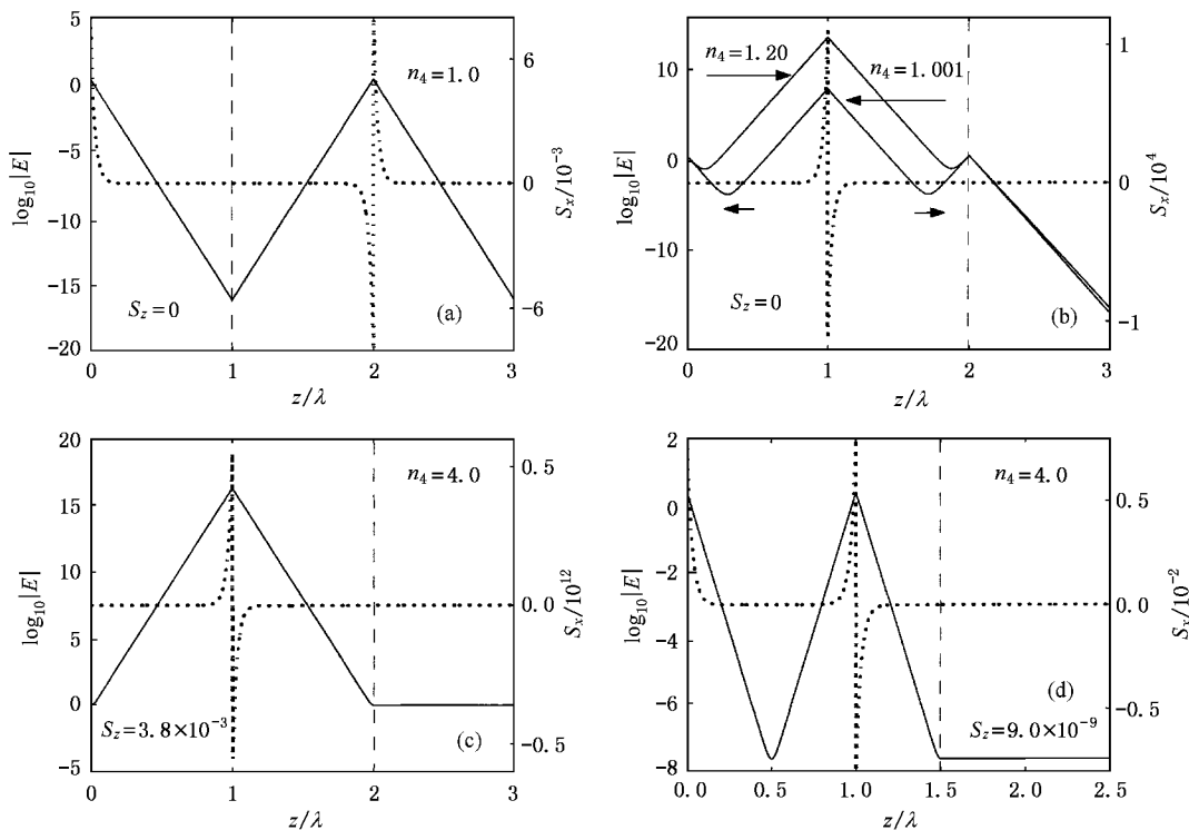
图 2 不同参数下的电场强度(实线)及沿 x 方向能流分布(点线)( k_x = 2\sqrt{2}k_0 , 细虚线表示不同介质区域的分界面)(a) d_2 = d_3 = \lambda 且阻抗匹配 n_4 = 1.0 (b) d_2 = d_3 = \lambda 且 n_4 分别为 1.001 和 1.20, 短箭头表示极小值移动的方向 (c) d_2 = d_3 = \lambda 且 n_4 = 4.0 (d) d_2 = 2d_3 = \lambda 且 n_4 = 4.0 . S_2 为常数,直接标注如图.注意(c)中远离跳变界面的 S_x 值为 \pm S_2 (远小于其跳变峰值)对应的能流方向为原 45^\circ 入射方向及其反常偏折的对称方向)
