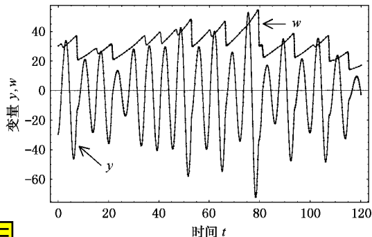
图4 本文方法(…)与 Runge-Kutta 法(—)计算方程(12)结果比较
