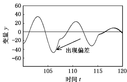
图3 外插4项时本文方法与 Runge-Kutta 法计算结果比较
