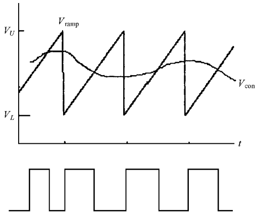
图 3 脉宽调制信号波形图
