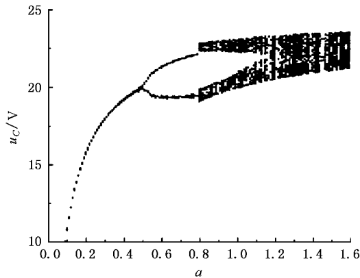
图 5 以反馈增益为分岔参数电压 u_C 的分岔图
