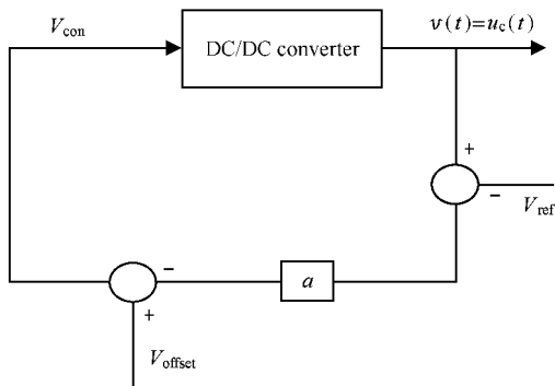
图 1 电压反馈型 DC-DC 变换器方框图
