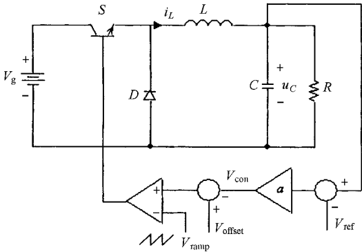
图 4 电压反馈型 buck 电路原理图
