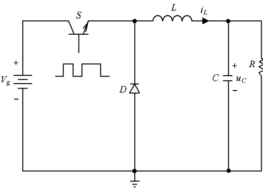
图 2 buck 变换器电路原理图
