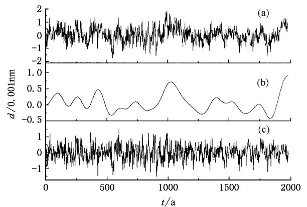
图 2 x(t) 的 100a 尺度滤波图像(横坐标为时间 t , 纵坐标为距平宽度 d )
