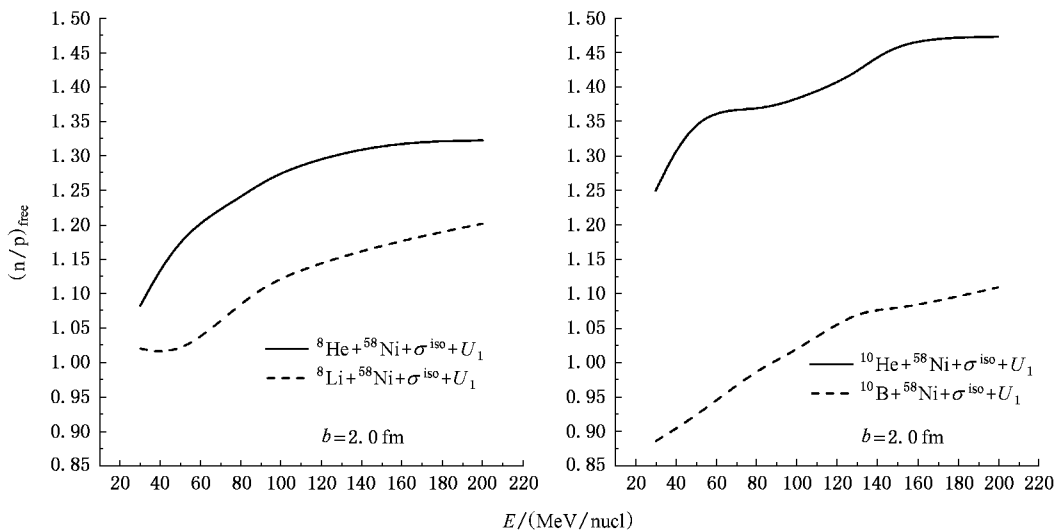
图 4 发射核子中子-质子比 \left(\frac{n}{p}\right)_{nucl} 随束流能量 E_b 的演化
