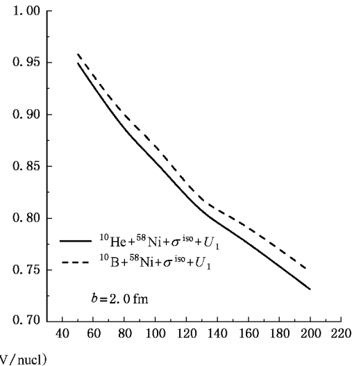
图 2 反应 ^8\text{He} + ^{58}\text{Ni} , ^8\text{Li} + ^{58}\text{Ni} , ^{10}\text{He} + ^{58}\text{Ni} 和 ^{10}\text{B} + ^{58}\text{Ni} 冻结时间原子核阻止 R 随束流能量 E_b 的演化
