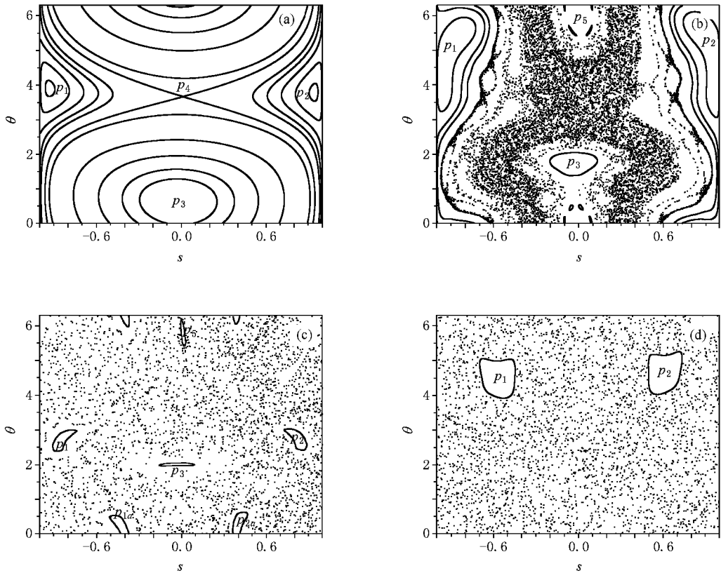
图 1 相平面中系统哈密顿量的演化 (a) c=0.3 (b) c=1.5 (c) c=2.2 (d) c=4.0
