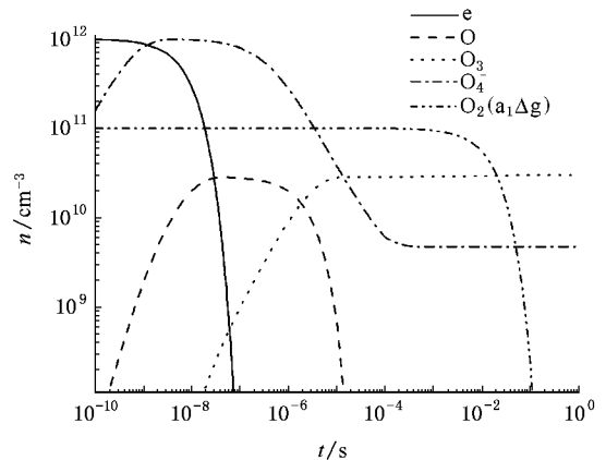
图 1 氧等离子体中主要组分随时间演化图
