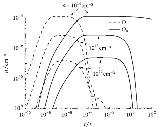
图4 大气等离子体不同电子初始数密度O和 O_3 随时间演化图 的形成过程,臭氧的最大数密度有限.为了加大生成臭氧的最大数密度,可以采用脉冲放电多次产生等离子体,形成高数密度臭氧.
