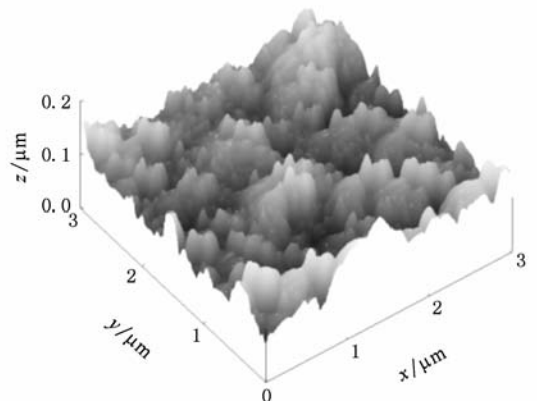
图4 镍磷黑吸收膜表面形貌图
