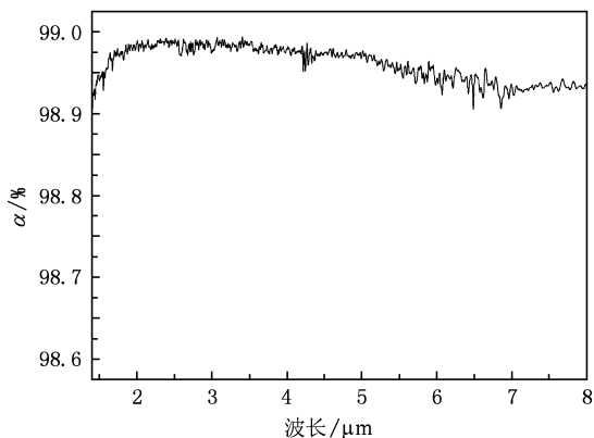
图5 镍磷黑吸收膜吸收率曲线
