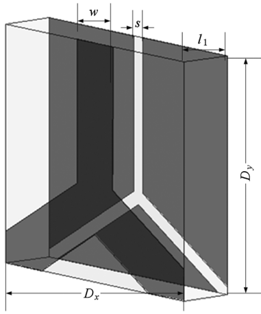
图3 MEFSS “Y”形周期单元及几何结构参数(阴影区域为金属)
