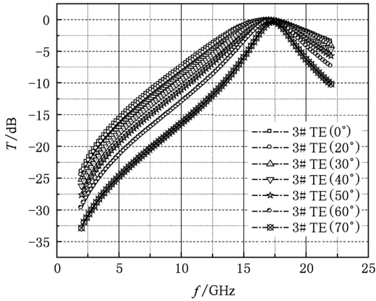
图 8 3#MEFSS 设计 TE 极化下不同入射角度时频率响应
