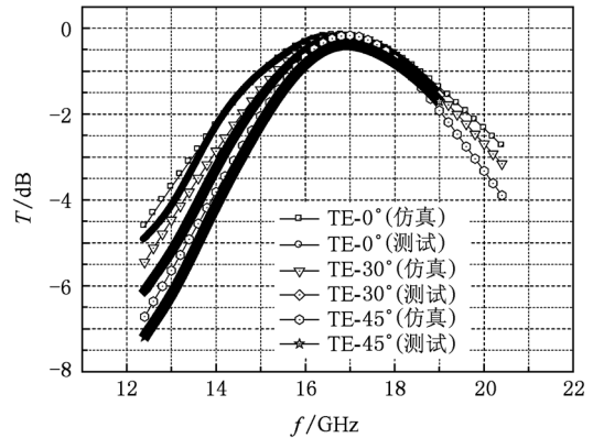
图 11 TE 极化 45°扫描仿真与测试
