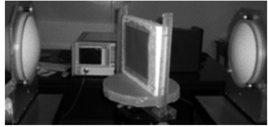
图 10 MEFSS 自由空间法测试系统
