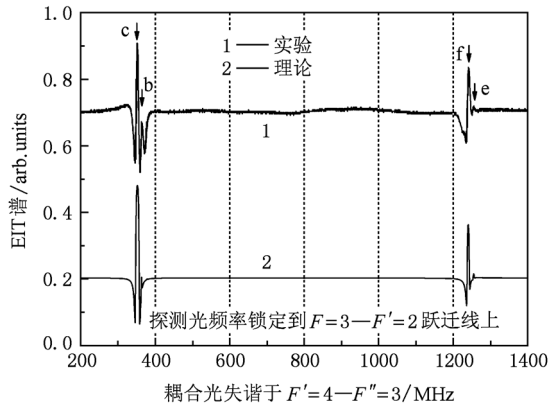
图 4 探测光频率锁定于 F=3-F'=2 跃迁线时的 EIT 谱
