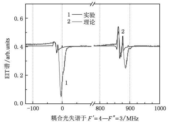
图 7 探测光频率锁定于 F=3-F'=4 跃迁线时的 EIT 光谱 (图 6 信号的放大)
