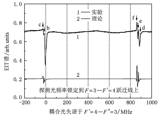
图 6 探测光频率锁定于 F=3-F'=4 跃迁线时的 EIT 光谱
