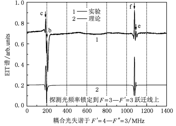
图 5 探测光频率锁定于 F=3-F'=3 跃迁线时的 EIT 谱
