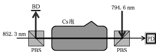
图 2 实验装置示意图(PBS:立方偏振棱镜;PD:光电探测器;BD:挡光板)
