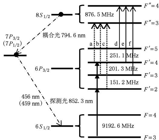
图 1 相关铯原子超精细能级图
