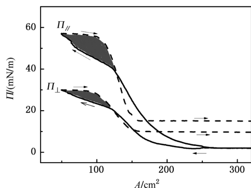
图 8 压缩-扩张循环中表面压的滞后现象
