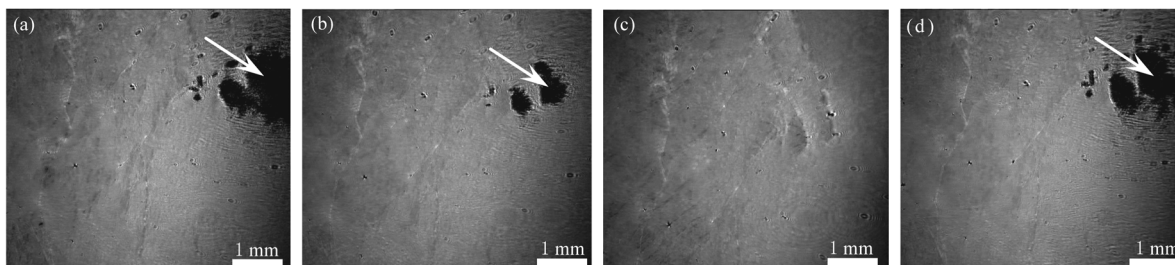
图7 高浓度膜( \Gamma = 50 \text{ mg/m}^2 )的形状记忆效应 (a) 孔洞尺寸减小; (b) 空洞尺寸减小; (c) 孔洞消失, \Gamma = 30 \text{ mg/m}^2 ; (d) 再次压缩后孔洞再现
