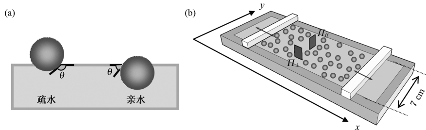
图 1 实验材料和实验装置示意图 (a) 润湿性不同的纳米颗粒在水面的吸附状态; (b) 配有两个互相垂直的 Wilhelmy 片的 Langmuir 槽
