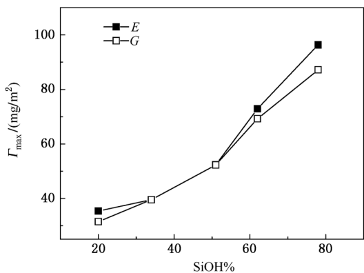
图5 \Gamma_{\max} 与纳米颗粒表面SiOH含量的关系
