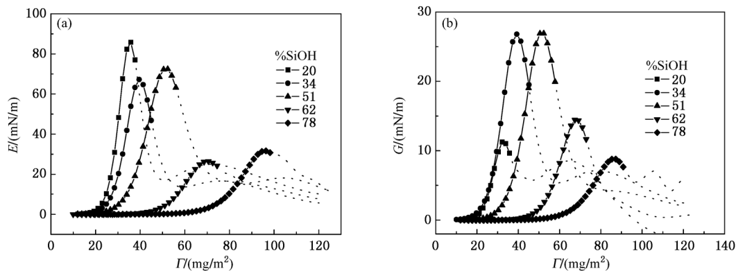
图4 不同润湿性纳米颗粒单层膜的模量 (a) E 与 \Gamma 的关系; (b) G 与 \Gamma 的关系
