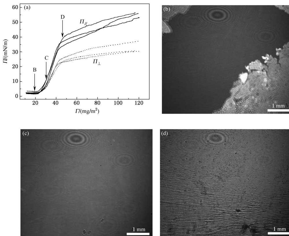
图 2 水/空气界面上 SiO 2 纳米颗粒(20% SiOH)单层膜表面压的各向异性及形貌演变 (a) \Pi - \Gamma 曲线, 压缩速率为 7 cm 2 /min, 实线为 \Pi_{//} ; 虚线为 \Pi_{\perp} ; (b)—(d) 分别为(a)中 B—D 点对应的 BAM 照片
