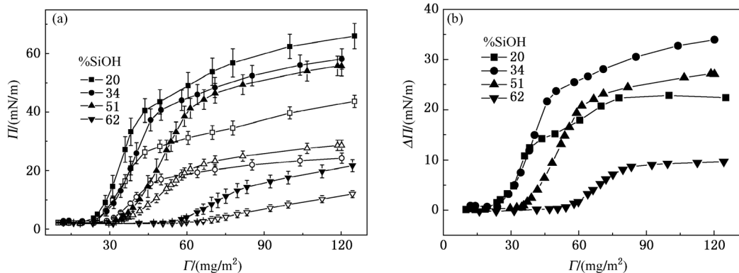
图3 不同润湿性纳米颗粒单层膜的表面压(压缩速率为 7 \text{ cm}^2/\text{min} ) (a) \Pi - \Gamma 曲线, 实心点为 \Pi_{\parallel} , 空心点为 \Pi_{\perp} ; (b) \Delta\Pi 与 \Gamma 的关系
