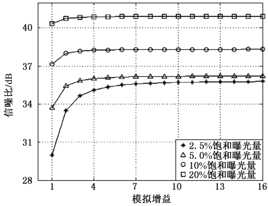
图5 不同曝光程度下模拟增益与信噪比的关系
