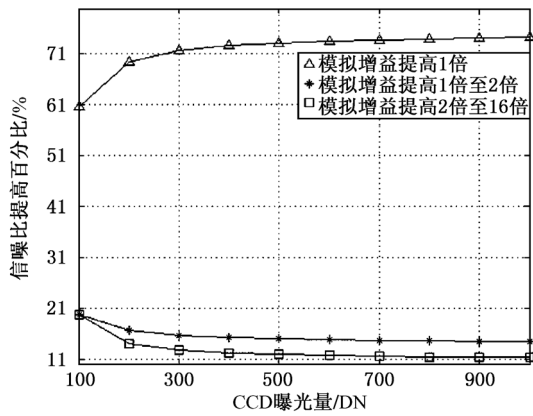
图6 模拟增益与信噪比提高百分比之间的关系
