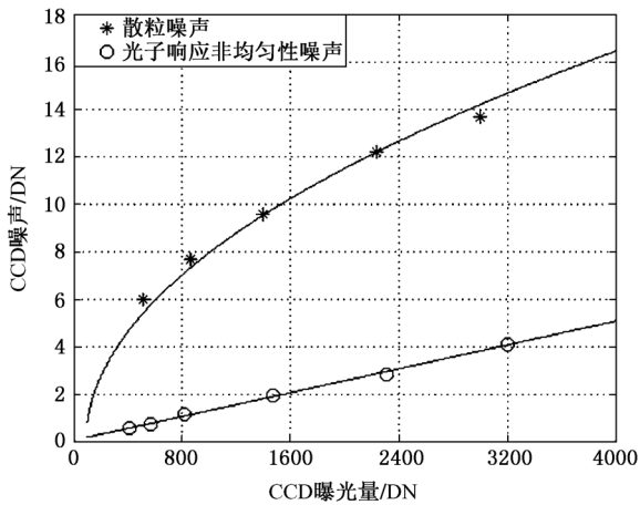
图3 CCD 噪声实验结果与拟合曲线
