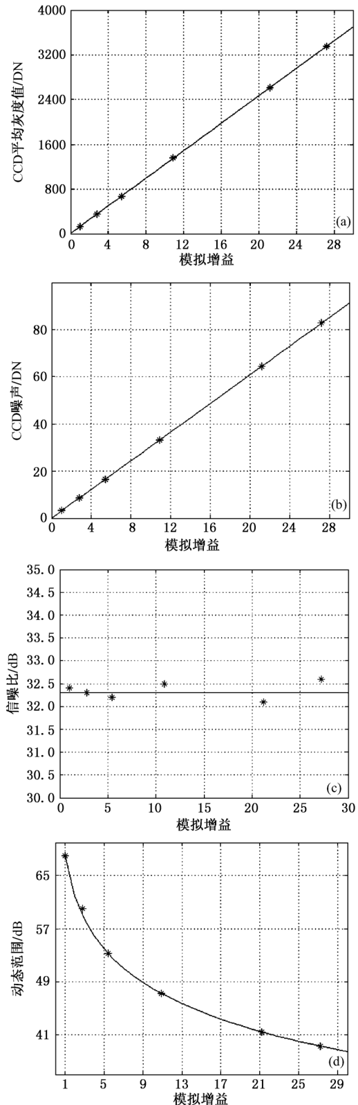
图4 模拟增益与(a)CCD 平均灰度值、(b) CCD 噪声、(c)信噪比、(d) 动态范围之间的关系
