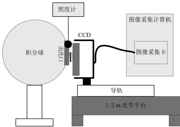
图 2 积分球标定实验原理框图
