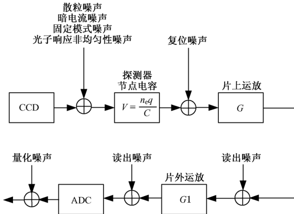
图 1 CCD 噪声源
