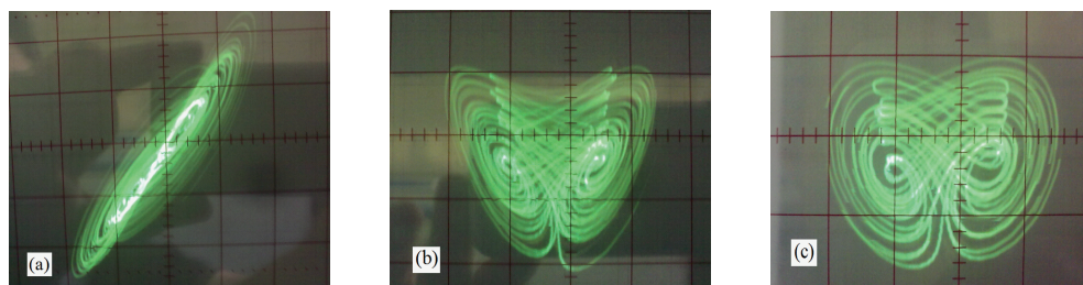
图 14 混沌系统 (1) 的电路实验结果 (a) x_1-x_2 平面; (b) x_1-x_3 平面; (c) x_2-x_3 平面
