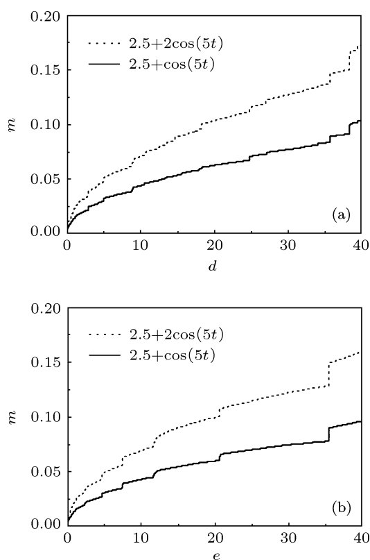
图 12 系统 (1) 中调幅度随不同参数的变化 (a) 参数 d ; (b) 参数 e
