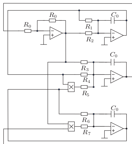
图 13 电路原理图
