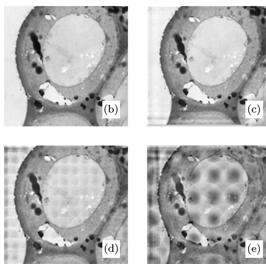
图 2 无移动偏差且重叠度为 60% 时挡板大小和入射光斑尺寸对重建图像质量的影响 (a) 不同尺寸入射探针条件下挡板大小对重建图像误差 RMS 的影响,图中还包括了单次平面波 CDI 的结果以作对比; (b) 测试原图: 苔藓细胞 SEM 图; (c)—(e) 为挡板半径 r_{\text{beamstop}} = 50 \text{ CCD 像素 (cps)} 时,探针直径 d_{\text{probe}} 分别为 28, 44 和 55 物空间像素 (fps) 时的重建图像. 它们的对应 RMS 值已在图 2(a) 中标出
