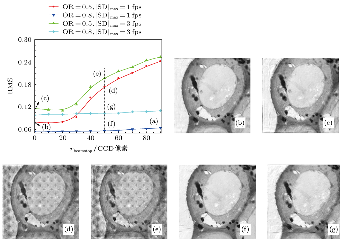
图 4 入射探针 d_{\text{probe}} = 55 \text{ fps} , 不同的移动偏差和探针重叠度条件下, 挡板大小对扫描相干衍射成像质量的影响 (a) 两种不同探针重叠度及移动偏差时挡板尺寸对 PCDI 重建误差的影响; (b)–(g) 不同参数下 PCDI 的重建图像, r_{\text{bs}} 表示挡板半径, 各图对应的 RMS 值已在图 (a) 中标出
