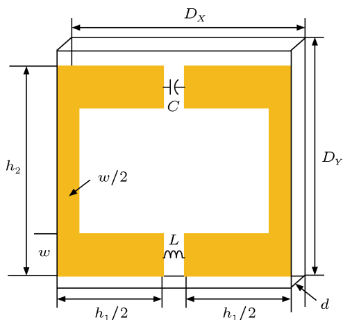
图 4 FSS 周期单元结构图
