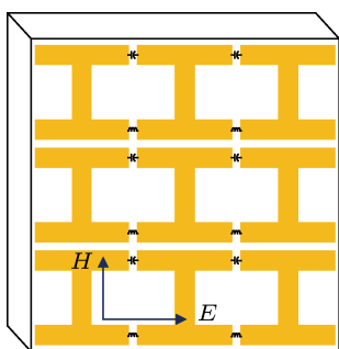
图 1 基于集总 LC 加载的 MEFSS 结构示意图
