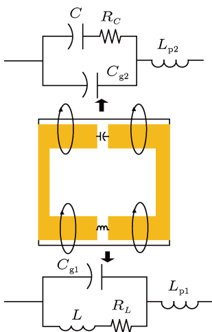
图 2 周期单元作用机理
