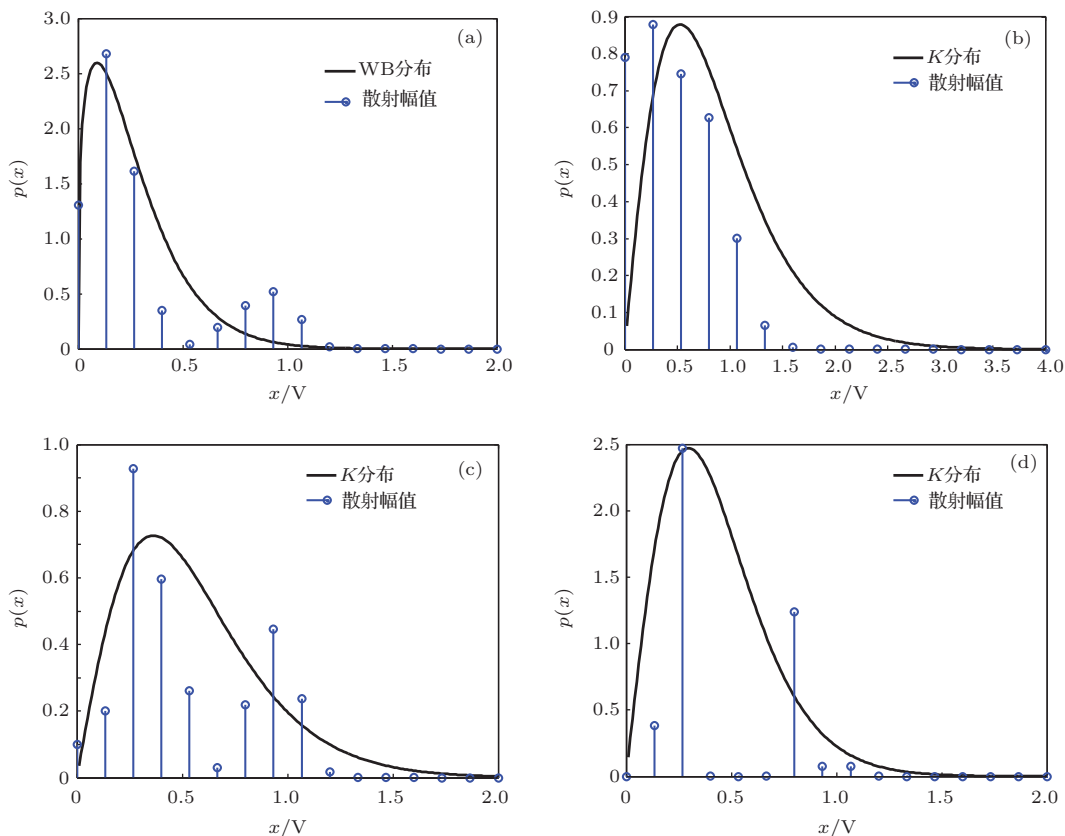
图4 逆风向85°入射时卷浪模型后向散射归一化幅值PDF及其拟合分布 (a) u = 10\text{ m}\cdot\text{s}^{-1} , HH极化; (b) u = 10\text{ m}\cdot\text{s}^{-1} , VV极化; (c) u = 15\text{ m}\cdot\text{s}^{-1} , HH极化; (d) u = 15\text{ m}\cdot\text{s}^{-1} , VV极化
