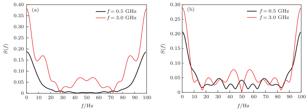
图6 (网刊彩色) 逆风入射角为 85^\circ 时, 不同入射频率下卷浪模型的后向散射多普勒谱 (a) 逆风, HH 极化; (b) 逆风, VV 极化
