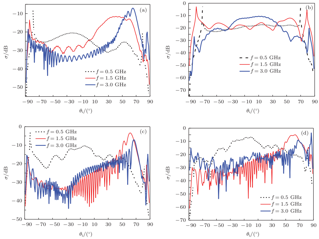
图2 (网刊彩色) 不同入射频率下卷浪模型后向散射系数角分布 (a) 第5条卷浪, HH 极化; (b) 第5条卷浪, VV 极化; (c) 第15条卷浪, HH 极化; (d) 第15条卷浪, VV 极化
