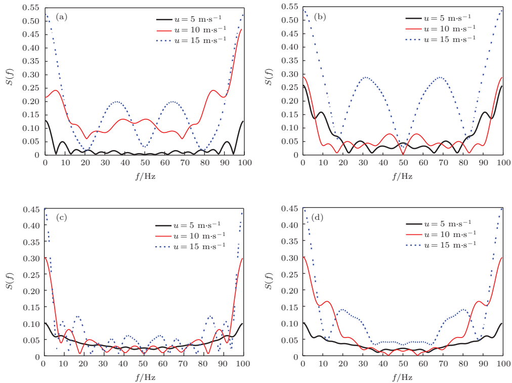
图5 (网刊彩色) 入射角为 85^\circ 时, 不同风速下卷浪模型后向散射多普勒谱 (a) 逆风, HH 极化; (b) 逆风, VV 极化; (c) 顺风, HH 极化; (d) 顺风, VV 极化
