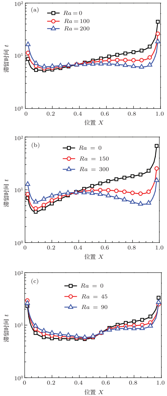
图4 非等温条件下滞留时间分布与Rayleigh 数的关系 (a)模型1; (b)模型2; (c)模型3
