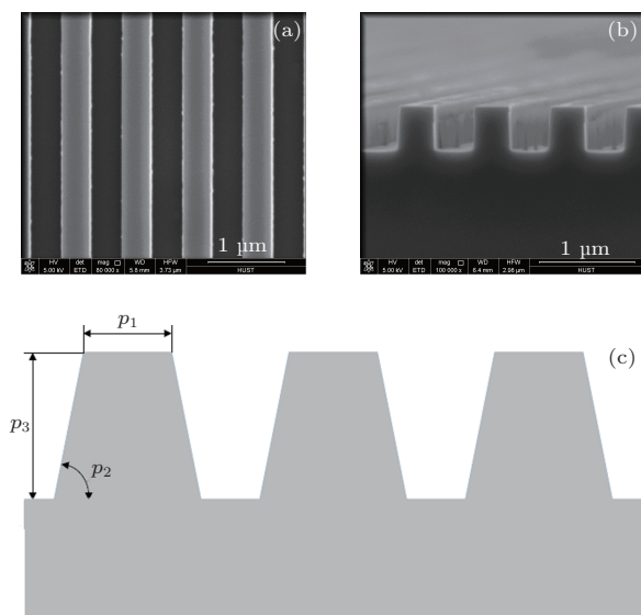
图 3 (a) 硅基光栅正面 SEM; (b) 硅基光栅侧面 SEM; (c) 光谱椭偏仪硅基光栅拟合模型
