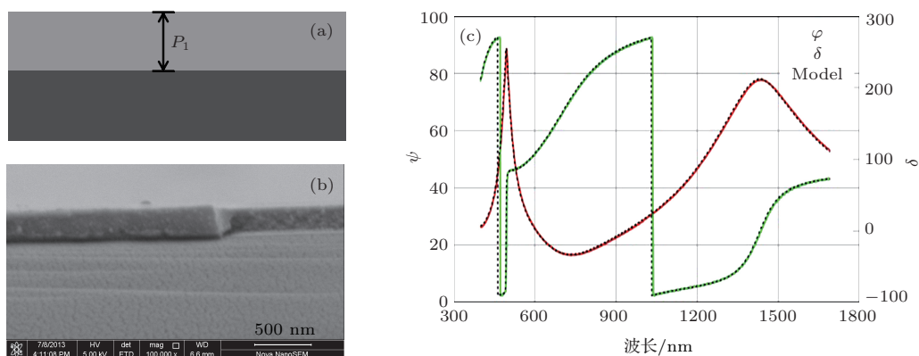
图2 (a) 拟合所建两层膜模型; (b) 硅基光刻胶 SEM; (c) 光谱椭偏仪拟合曲线
