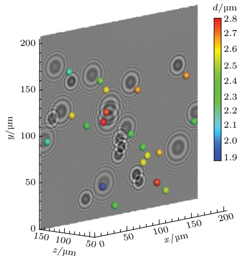
图8 (网刊彩色) d = 2-3 \mu\text{m} 的非透明颗粒场的模拟全息图和三维重建
