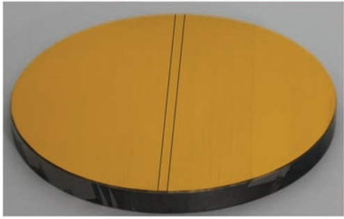
图 16 (网刊彩色) 低阶梯多级微反射镜 Fig. 16. (color online) Low stepped-mirror.
