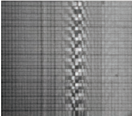
图 18 SiC 光源制冷时的干涉图 Fig. 18. Interferogram of cold light source.
