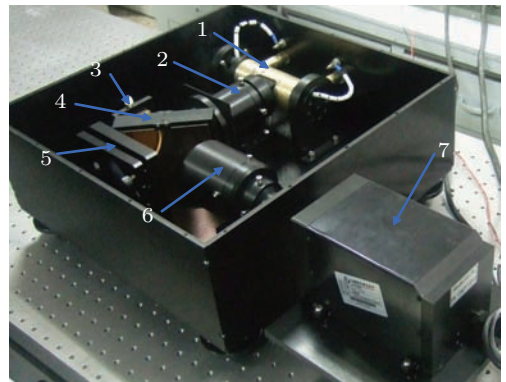
图 14 (网刊彩色) 系统结构图 1 光源; 2 准直系统; 3 高阶阶梯多级微反射镜; 4 分束系统; 5 低阶梯多级微反射镜; 6 缩束系统; 7 红外探测器
