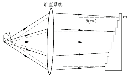
图5 存在离焦时准直系统子午光线在不同阶梯上的入射角示意图
