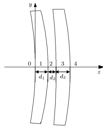
图 2 准直系统结构示意图
