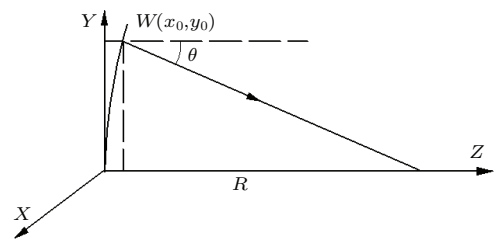
图6 准直系统离焦时出瞳面上的球面波前
