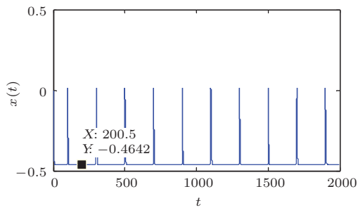
图 7 脉冲信号平移后的单稳系统响应
