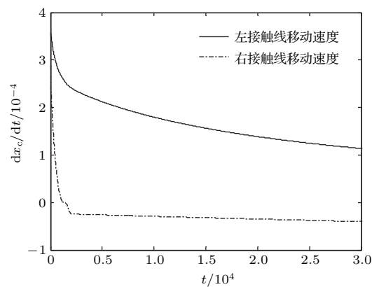
图 8 液滴两侧接触线的移动速度 ( \Gamma = 0.02 , \Sigma_{ls} = 1.01 , \Sigma_{sg} = \Sigma_{lg} = 1.0 )
