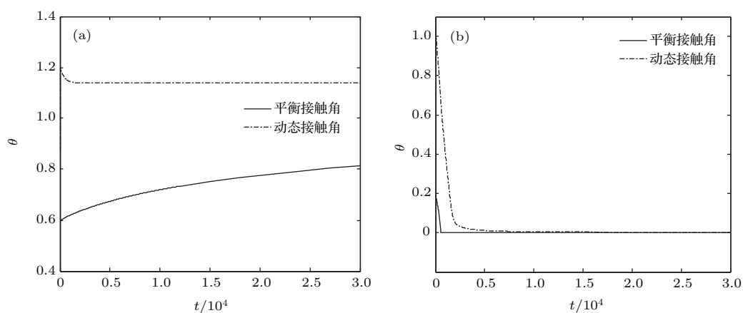
图 10 两侧接触角的变化 ( \Gamma = 0.02 , \Sigma_{ls} = 1.04 , \Sigma_{sg} = \Sigma_{lg} = 1.0 ) (a) 左侧接触角; (b) 右侧接触角
