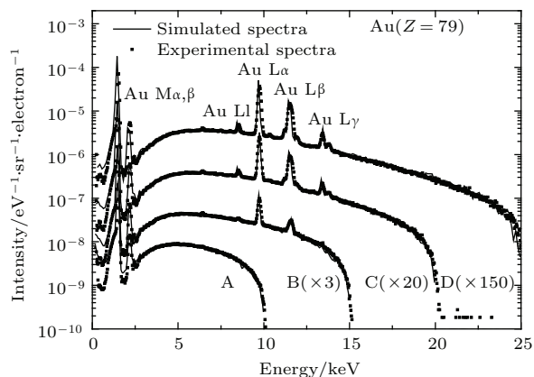
图2 由(A) 10, (B) 15, (C) 20, (D) 25 keV电子碰撞厚Au靶产生的韧致辐射实验谱与PENELOPE模拟谱的对比. 点表示实验谱, 实线表示模拟谱; 为了实验谱和模拟谱的清晰对比, B, C, D分别乘以括号中的系数.
