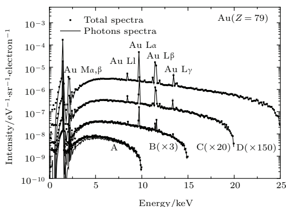
图4 PENELOPE模拟(A) 10, (B) 15, (C) 20, (D) 25 keV电子碰撞Au靶产生的能量谱中光子和电子的总贡献与光子贡献的比较. 点表示光子和电子的总贡献谱, 实线表示光子的贡献谱; 为了清晰, B, C, D分别乘以括号中的系数.
