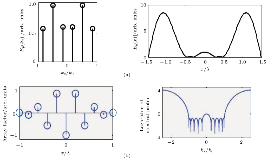
图 5 超振荡与超方向 (a) 超振荡. 左为空间频谱, 右为其对应的超振荡波形 (空间域); (b) 超方向. 左为阵列因子, 右为其对应的超振荡频谱 (空间频域)
