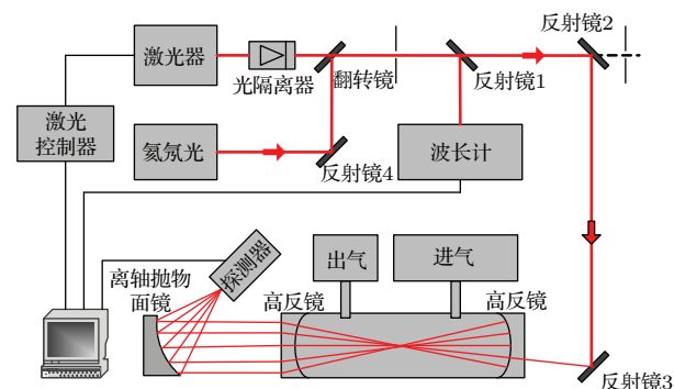
图1 离轴积分腔实验装置简图
