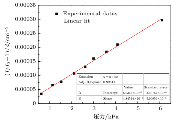
图6 腔体里面 \text{CH}_4 压力与积分面积之间的关系
