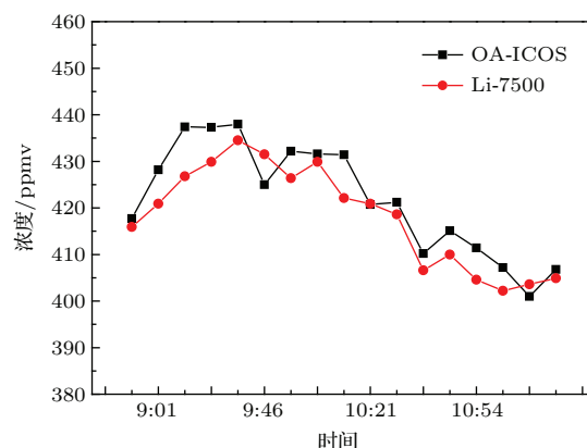
图8 两套装置测量得到的 \text{CO}_2 浓度对比及其随时间的变化
