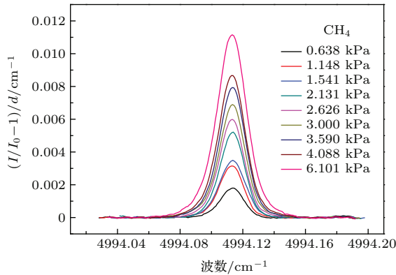
图5 (网刊彩色) 不同压力下 \text{CH}_4 吸收谱线的变化
