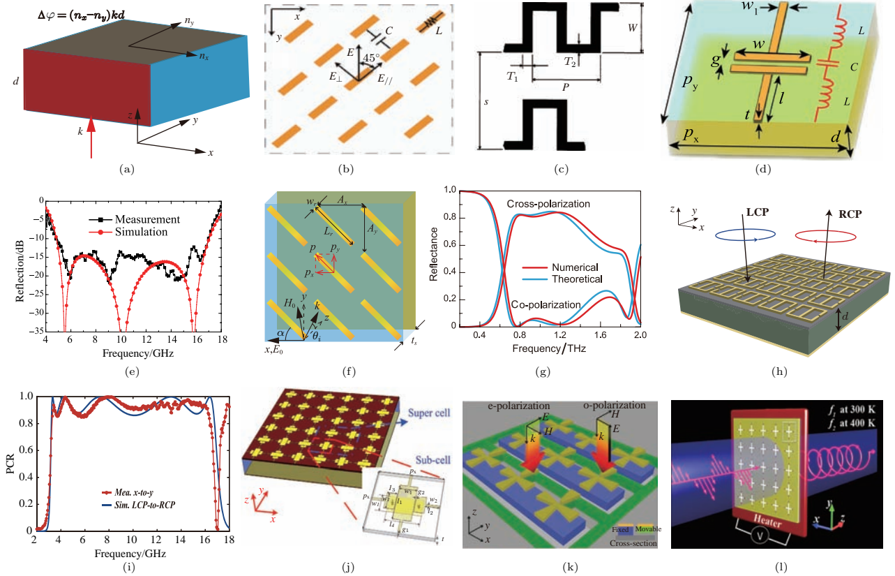
图9 各向异性亚波长结构偏振调控材料 (a)各向异性结构的偏振调制原理示意图;(b)金属线结构亚波长偏振调控材料结构示意图;(c)基于曲折线结构的偏振调控材料[109];(d),(e)分别为基于工字形的宽带偏振调控亚波长结构及主偏振反射曲线[101];(f),(g)分别为基于金属线结构的太赫兹偏振调控器件及主偏振和交叉偏振反射率曲线[106];(h),(i)分别为基于二维色散调控的超宽带偏振调控材料及其偏振转换效率曲线[110];(j)微波波段各向异性偏振动态调控亚波长结构材料[111];(k)基于微机械系统的偏振动态调控亚波长结构材料[112];(l)基于相变材料的太赫兹偏振动态调控亚波长结构材料[113]
