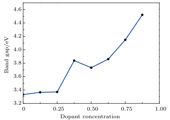
图4 \text{Zn}_{1-x}\text{Ba}_x\text{O} 禁带宽度与原子掺杂百分比的关系 Fig. 4. Dependence of band gap versus dopant percentage.
