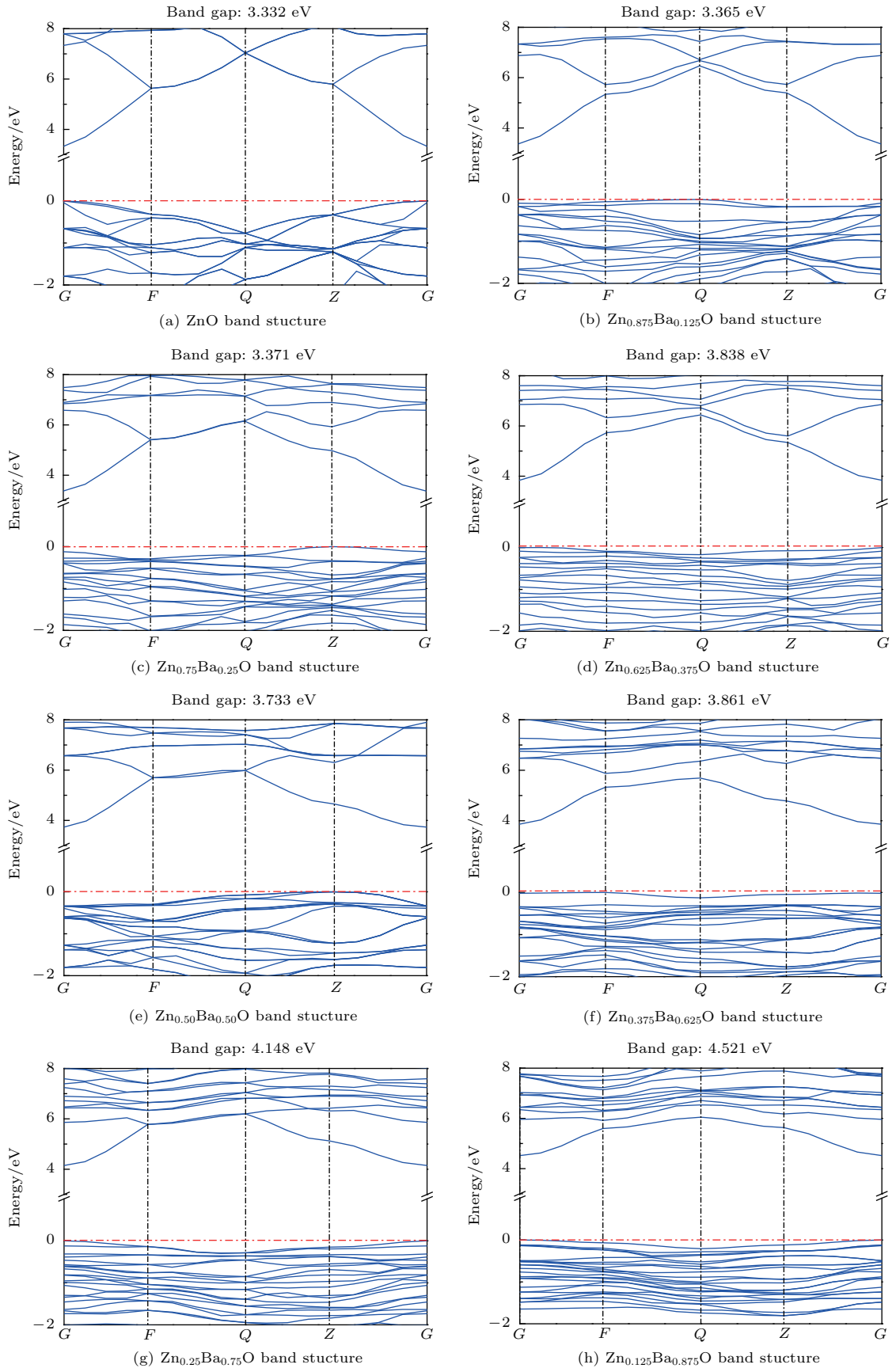
图3 \text{Zn}_{1-x}\text{Ba}_x\text{O} 的能带结构
