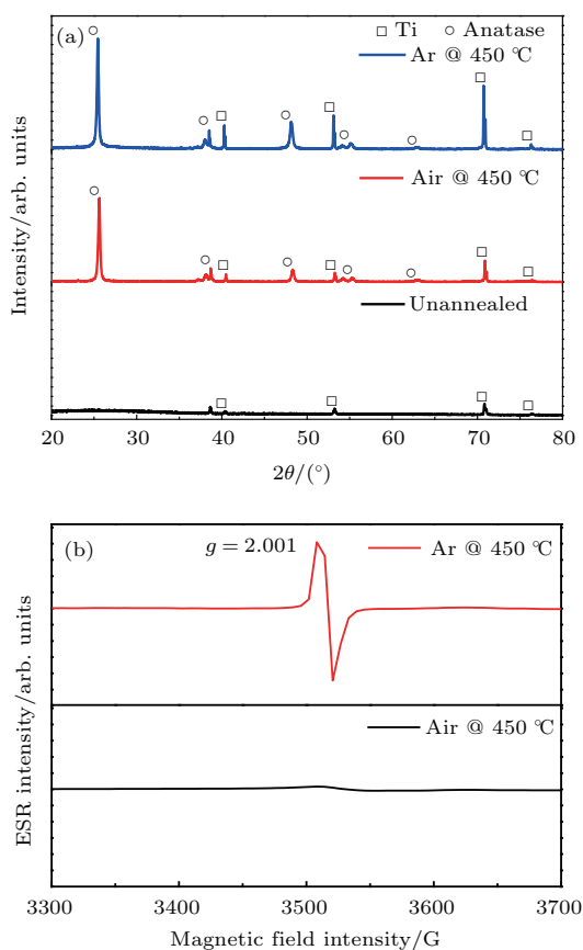
图3 未退火样品、空气和氩气氛围下退火样品的 TNTAs 薄膜的 (a) XRD 图谱和 (b) ESR 图谱
