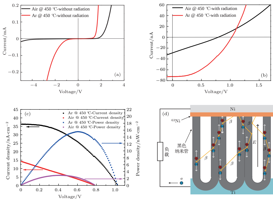
图5 (a) 空气退火和氩气退火样品未应用辐射源结构 (Ni/TNTAs/Ti) 的 I - V 特性; (b) 空气退火和氩气退火样品应用辐射源结构 ( ^{63}\text{Ni} /TNTAs/Ti) 的 I - V 特性; (c) 空气退火和氩气退火样品同位素电池的电流密度曲线和功率密度曲线; (d) 基于一维 TNTAs 薄膜的 ^{63}\text{Ni} 同位素电池结构示意图
