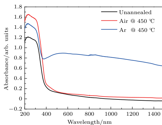
图4 未退火样品、空气和氩气氛围下退火样品的 TNTAs 薄膜的紫外-可见光吸收光谱
