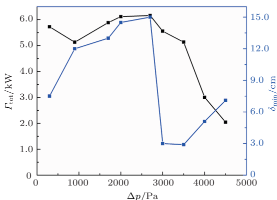
图9 不同 \Delta p 下钝体表面总热流密度和包覆钝体头部的等离子体鞘套最小厚度的变化规律
