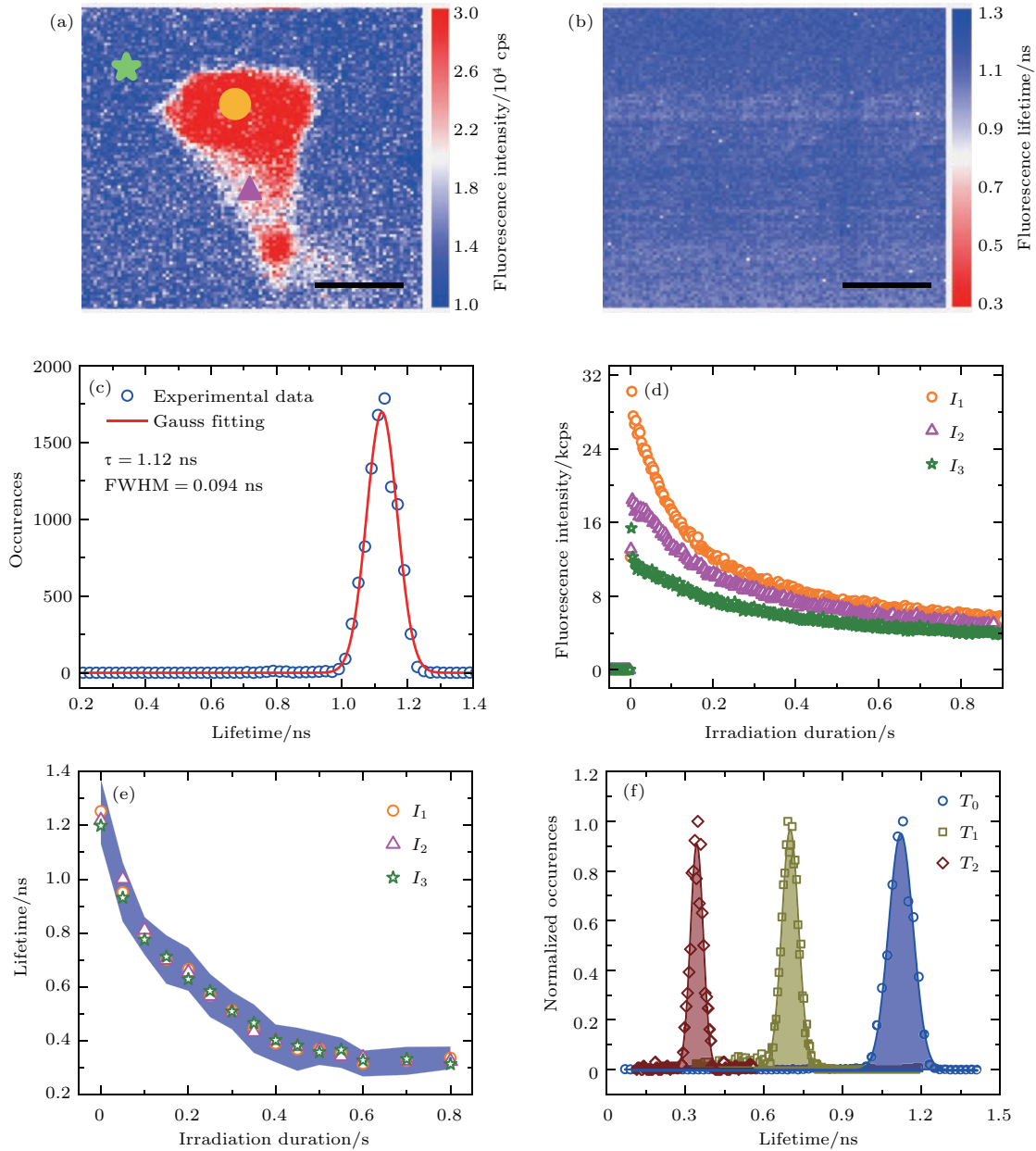
图3 (a), (b) GO薄膜的荧光强度成像和寿命成像, 比例尺 10 \mu\text{m} ; (c) 寿命分布统计; (d), (e) 分别为图(a)中三处标记位置荧光强度和荧光寿命随 405 nm 激光照射时间的衰减情况, 激光功率为 1.5 mW, (e) 蓝色条形为寿命误差; (f) 未还原 ( T_0 )、还原 0.1 s ( T_1 ) 和还原 0.5 s ( T_2 ) 后其荧光寿命的统计分布, 在 T_0 , T_1 , T_2 下, 寿命分别为 (1.122 \pm 0.047) ns, (0.700 \pm 0.031) ns, (0.343 \pm 0.024) ns
