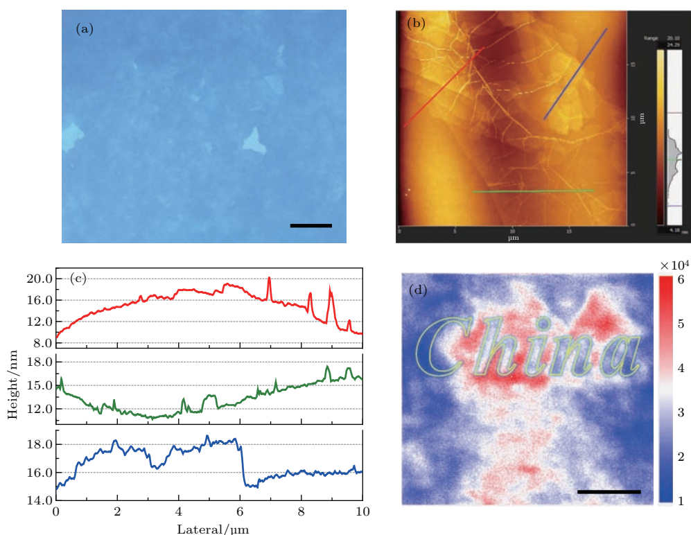
图2 (a), (b) 分别为GO薄膜的光学成像和原子力显微成像,比例尺10 \mu\text{m} ; (c) 为(b)图中两点连线方向样品高度的剖面图; (d) GO薄膜荧光强度成像图,图中标记“China”区域为405 nm激光还原部分,比例尺10 \mu\text{m}
