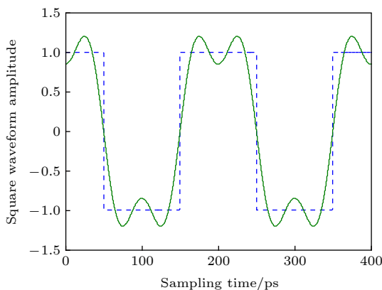
图 2 \beta = 2.30 时生成的三阶方波 (实线) 与理想方波 (虚线) 的波形图
