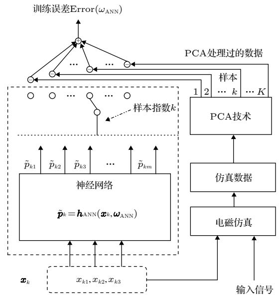
图 1 结合 PCA 技术的神经网络模型结构
