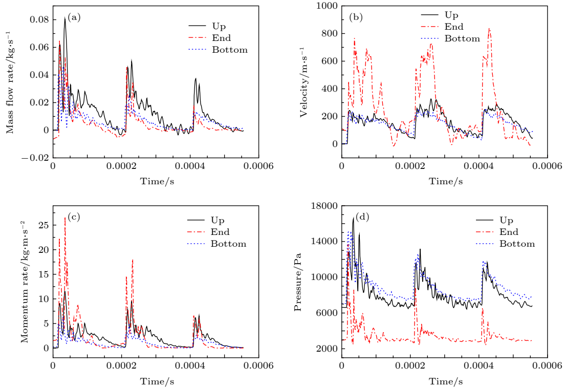
图 18 激励器出口参数 (a) 激励器出口质量流量; (b) 激励器出口速度; (c) 激励器出口动量率; (d) 激励器出口压力 Fig. 18. The parameters of actuator outlet: (a) The mass flow rate of actuator outlet; (b) the velocity of actuator outlet; (c) the momentum rate of actuator outlet; (d) the pressure of actuator outlet.
