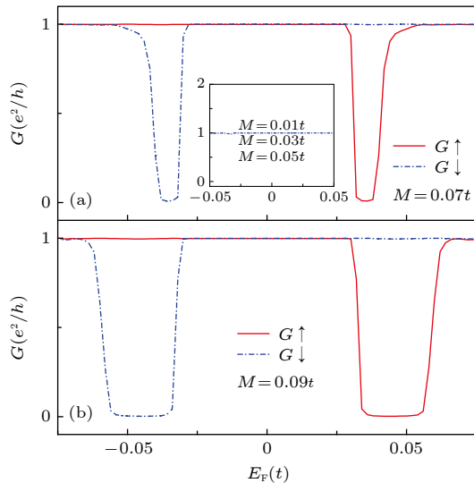
图 2 施加不同强度的局域交换场 M 时, 电导 G 与电子费米能量 E_F 之间的关系 (红色实线表示自旋向上的电子, 蓝色虚线表示自旋向下的电子) (a) M = 0.01t, 0.03t, 0.05t, 0.07t 时的自旋相关电导; (b) M = 0.09t 时的自旋相关电导
