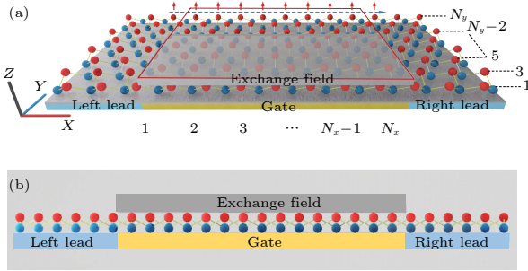
图 1 (a) 单层锗烯自旋过滤器件结构示意图 (左、右两侧蓝色区域为左、右电极区域; 中间红色实线包围区域为中心器件区; 灰色和黄色分别表示 Z 轴方向交换场和电场的施加区域); (b) 单层锗烯自旋过滤器件侧视图 (红色和蓝色小球分别代表锗烯翘曲层顶部和底部的锗原子)
