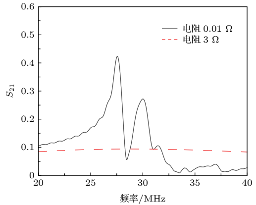
图 9 贴片电容与电阻串联时的仿真效率
