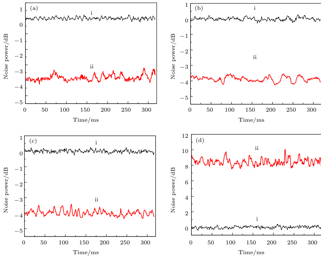
图 3 偏振压缩光 Stokes 分量的量子噪声 [61] (a) \hat{S}_0 ; (b) \hat{S}_1 ; (c) \hat{S}_2 ; (d) \hat{S}_3
