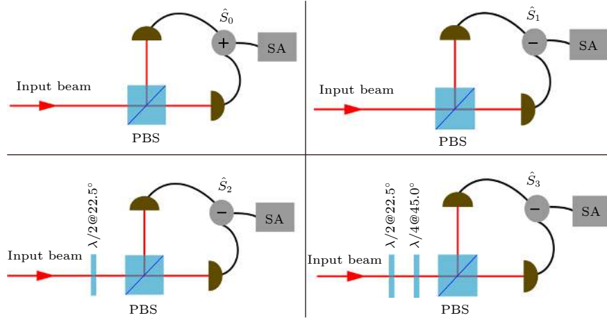
图 2 四个斯托克斯参数的测量装置. PBS, 偏振分束棱镜; \lambda/2 和 \lambda/4 分别是半波片和四分之一波片; 加号和减号分别代表电流信号相加减; SA, 频谱分析仪
