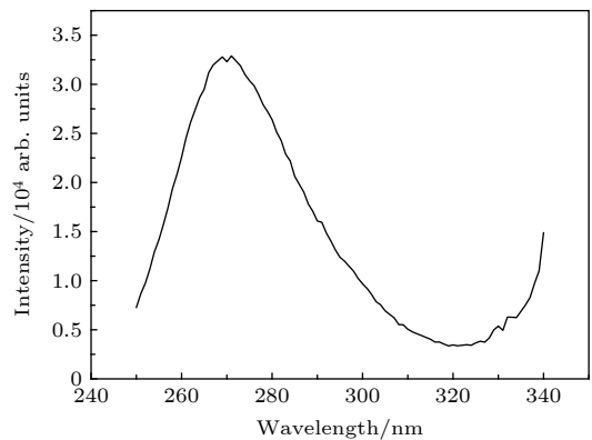
图 8 退火前后 Ti:MgAl_2O_4 晶体 480 nm 发射的激发光谱
