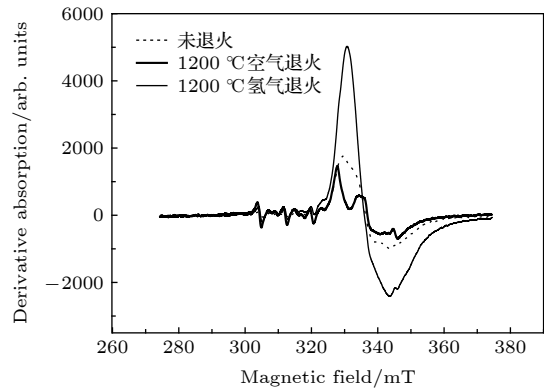
图 7 Ti:MgAl_2O_4 晶体在 130 K 时的 ESR 谱
