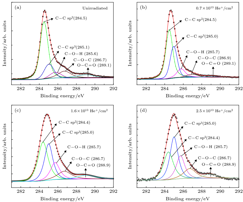
图 1 石墨烯样品 XPS C 1s 峰谱图 (a) 未辐照; (b) 0.7 × 10 13 He + /cm 2 ; (c) 1.6 × 10 13 He + /cm 2 ; (d) 2.5 × 10 13 He + /cm 2
