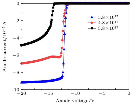
图 9 不同掺杂浓度下肖特基二极管反向 I - V 曲线 Fig. 9. Reverse I - V curves of Schottky diode under different doping concentrations.
