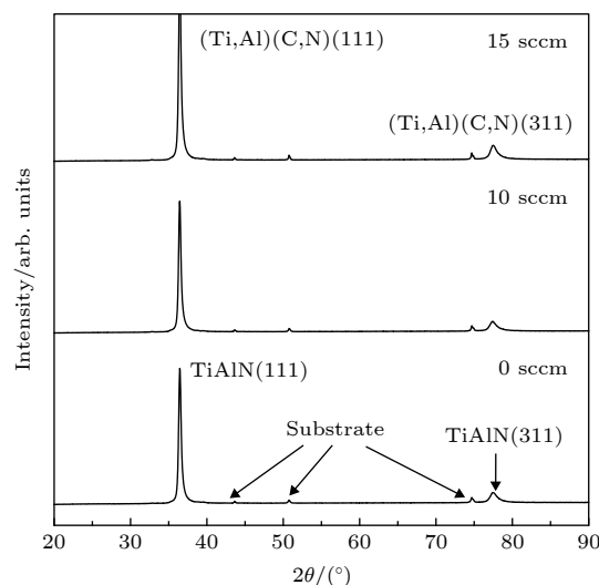
图 4 不同 \text{C}_2\text{H}_2 流量沉积的 TiAlCN/TiAlN/TiAl 涂层的 XRD 图谱
