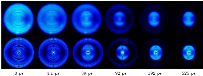
图 3 泵浦光 323 nm, 探测光 400 nm, 在不同时间延迟下的光电子原始影像和 BASEX 变换后的影像 (上排为原始影像, 而下排为 BASEX 变换后的影像). 泵浦光和探测光都是线偏振光, 偏振方向为图平面竖直方向
