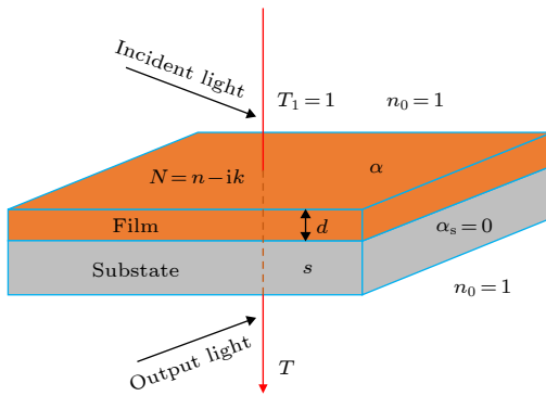
图 1 镀在透明二氧化硅玻璃衬底上的薄膜结构示意图 Fig. 1. Schematic of the structure of a thin film coated on a transparent silica glass substrate.
