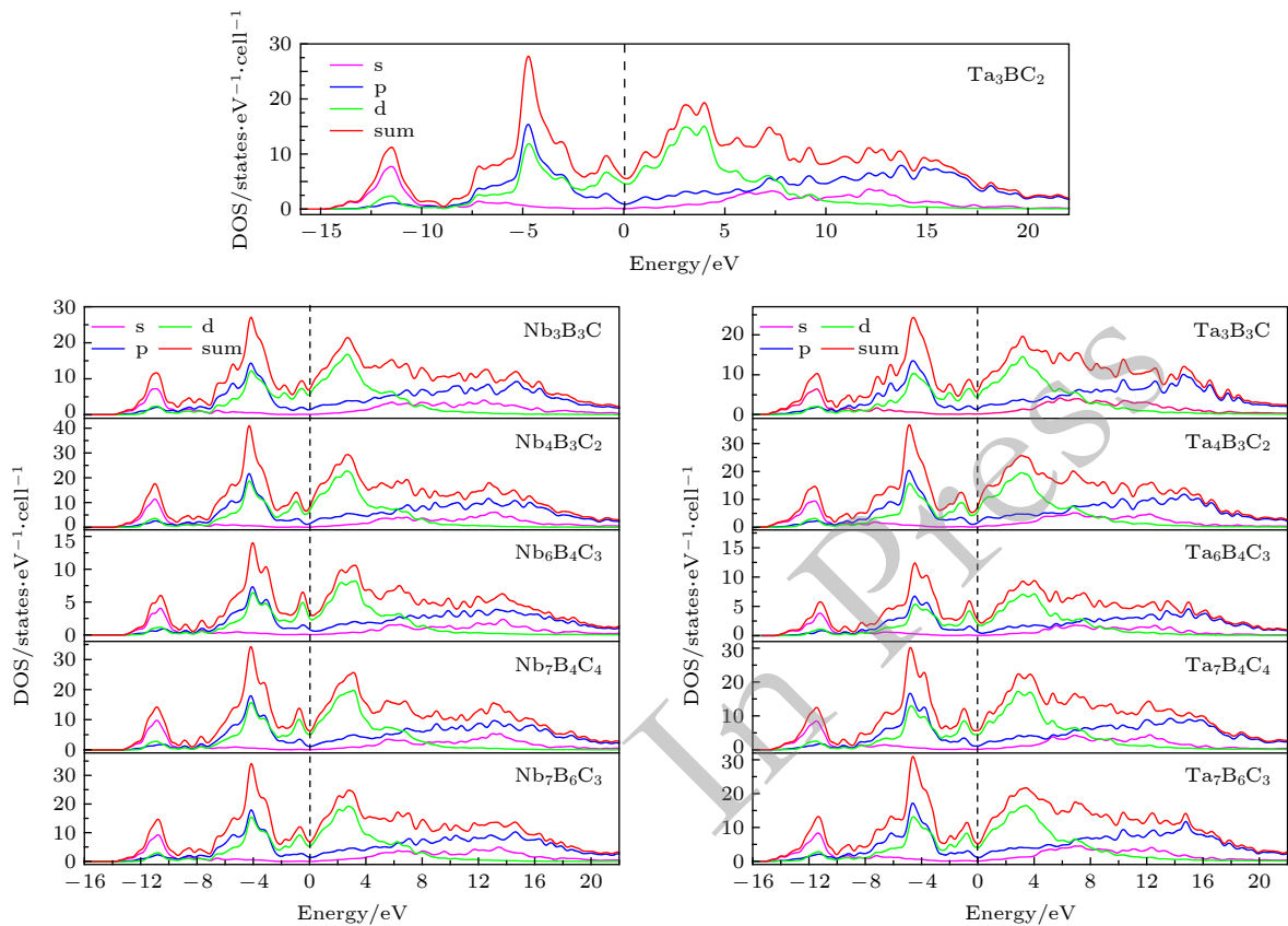
图 5 Nb-B-C 和 Ta-B-C 三元相的态密度图
