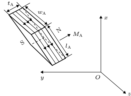
图 8 矩形磁铁尺寸及磁化电流示意图
