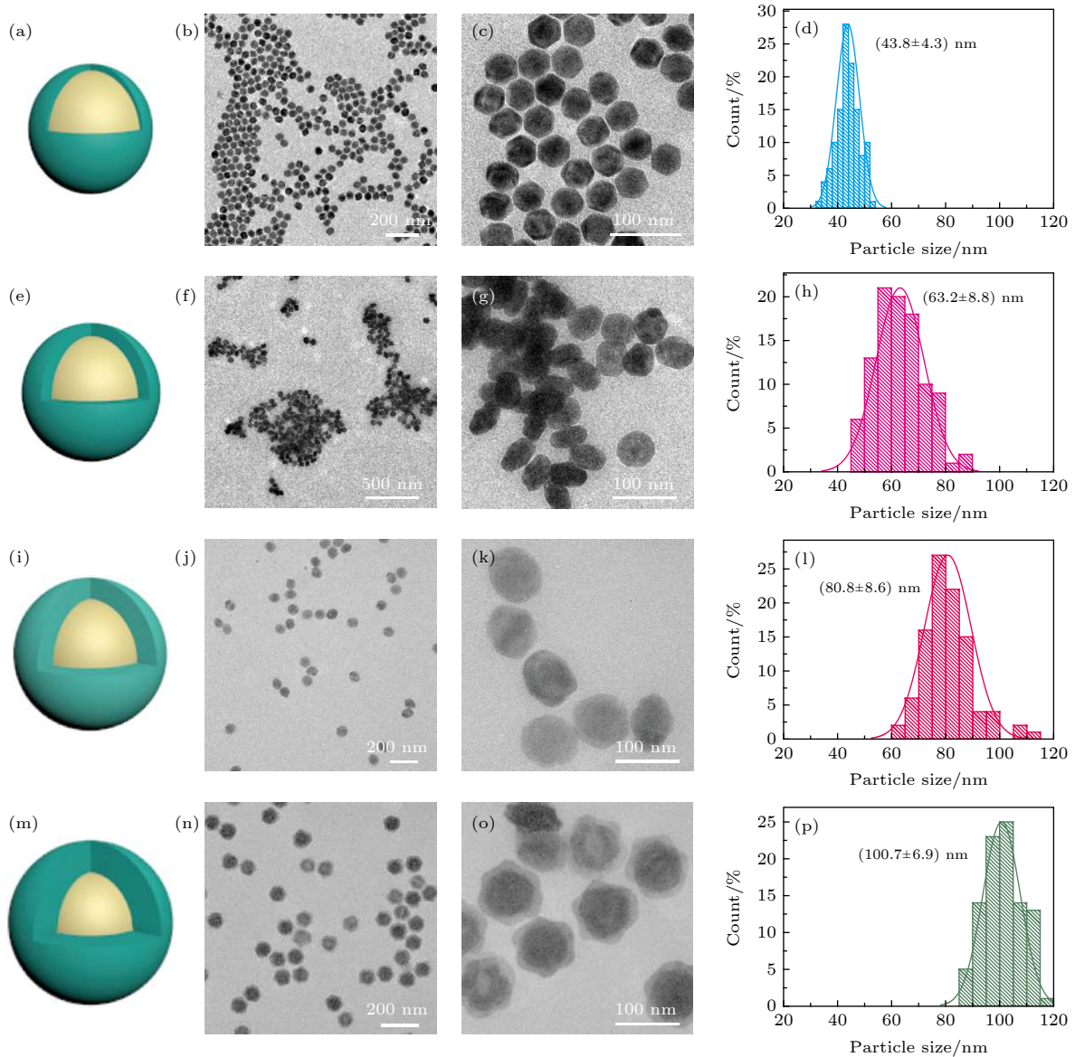
图3 (a)—(d) \text{NaYF}_4:\text{Yb, Tm}@\text{NaYF}_4 纳米粒子 (粒径约 43.8 nm) 的结构示意图, TEM 图和粒径分布图; (e)—(h) \text{NaYF}_4:\text{Yb, Tm}@\text{NaYF}_4 纳米粒子 (粒径约 63.2 nm) 的结构示意图, TEM 图和粒径分布图; (i)—(l) \text{NaYF}_4:\text{Yb, Tm}@\text{NaYF}_4 纳米粒子 (粒径约 80.8 nm) 的结构示意图, TEM 图和粒径分布图; (m)—(p) \text{NaYF}_4:\text{Yb, Tm}@\text{NaYF}_4 纳米粒子 (粒径约 100.7 nm) 的结构示意图, TEM 图和粒径分布图
