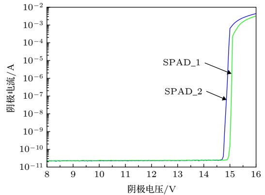
图 4 器件 I-V 特性曲线图
