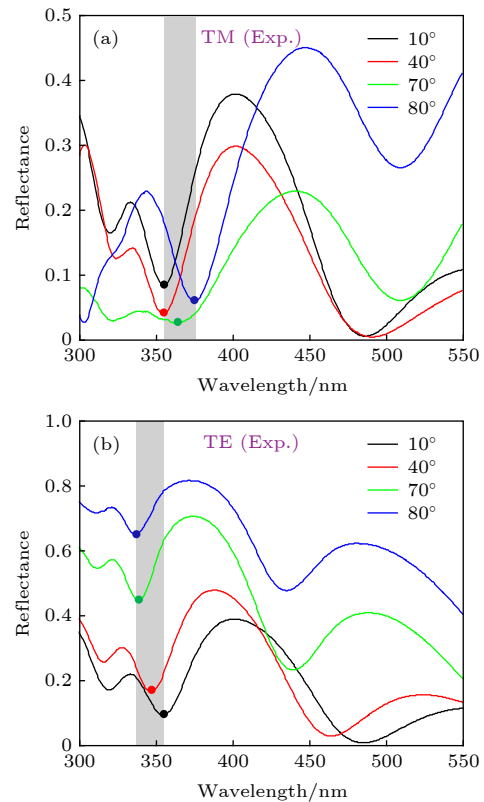
图 10 实验测量的含双曲超构材料的一维光子晶体 [(CD)^2B]^3 在不同入射角下的反射谱 (a) TM 偏振 [108] ; (b) TE 偏振 [108]
