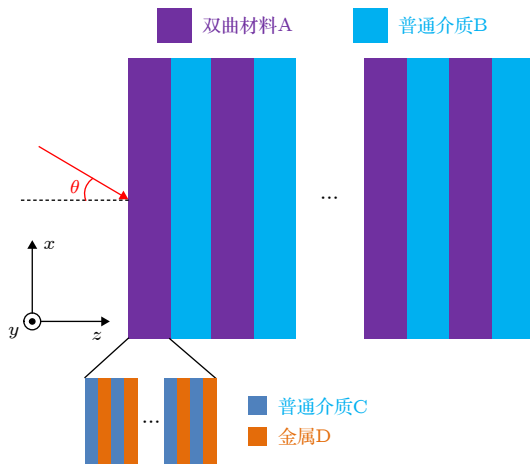
图 5 含双曲超构材料的一维光子晶体 [(CD)^S B]^N 的示意图
