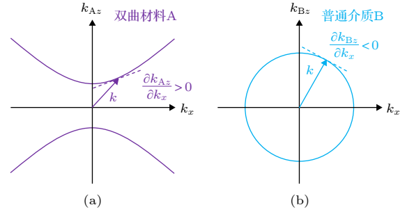
图 6 (a) 双曲材料 A 和 (b) 普通介质 B 的等频线 (TM 偏振)
