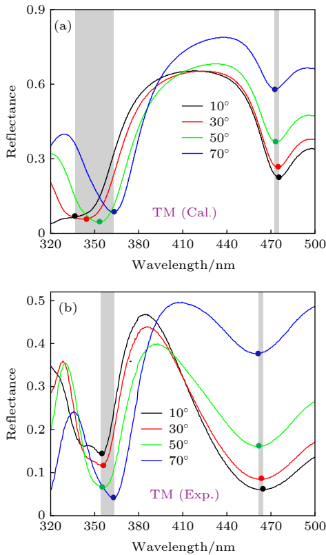
图 7 含双曲超构材料的一维光子晶体 [(\text{CD})^2\text{B}]^3 在不同入射角下的反射谱 (TM 偏振) (a) 数值计算结果 [107] ; (b) 实验测量结果 [107]
