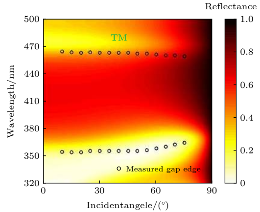
图 8 含双曲超构材料的一维光子晶体 [(\text{CD})^2\text{B}]^3 的反射谱 (TM 偏振) 随入射角的变化 [107] , 其中彩色背景代表数值计算结果, 黑色空心圆圈代表实验测量的带隙边缘 (由最靠近带隙的反射极小值提取)
