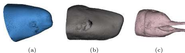
图 1 (a) 东亚江豚头部的三维重建; (b) 小抹香鲸头部的三维重建; (c) 中华白海豚头部的三维重建
