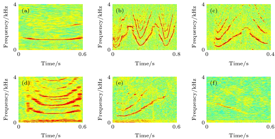
图 6 (a) 宽吻海豚固定频率型通信声信号时频图; (b) 宽吻海豚正弦型通信声信号时频图; (c) 宽吻海豚凸型通信声信号时频图; (d) 宽吻海豚凹型通信声信号时频图; (e) 宽吻海豚上扫频型通信声信号时频图; (f) 宽吻海豚下扫频型通信声信号时频图 [58,59] ; 其中颜色深浅表示声信号强度大小
