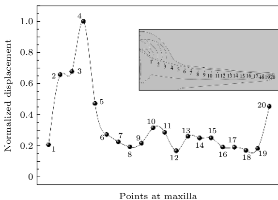
图 10 白黵豚上颌骨表面 20 个点的固体位移分布情况 [74]
