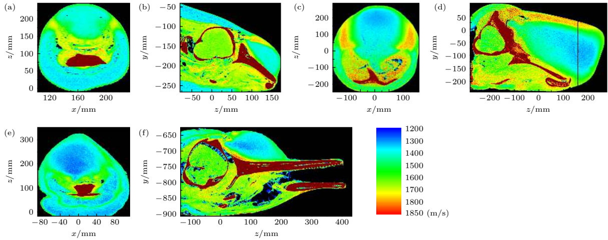
图3 (a) 东亚江豚头部声发射系统的水平截面声速重建; (b) 东亚江豚头部声发射系统的垂直截面声速重建 [34] ; (c) 小抹香鲸头部声发射系统的水平截面声速重建; (d) 小抹香鲸头部声发射系统的垂直截面声速重建 [36] ; (e) 中华白海豚头部声发射系统的水平截面声速重建; (f) 中华白海豚头部声发射系统的垂直截面声速重建 [38]
