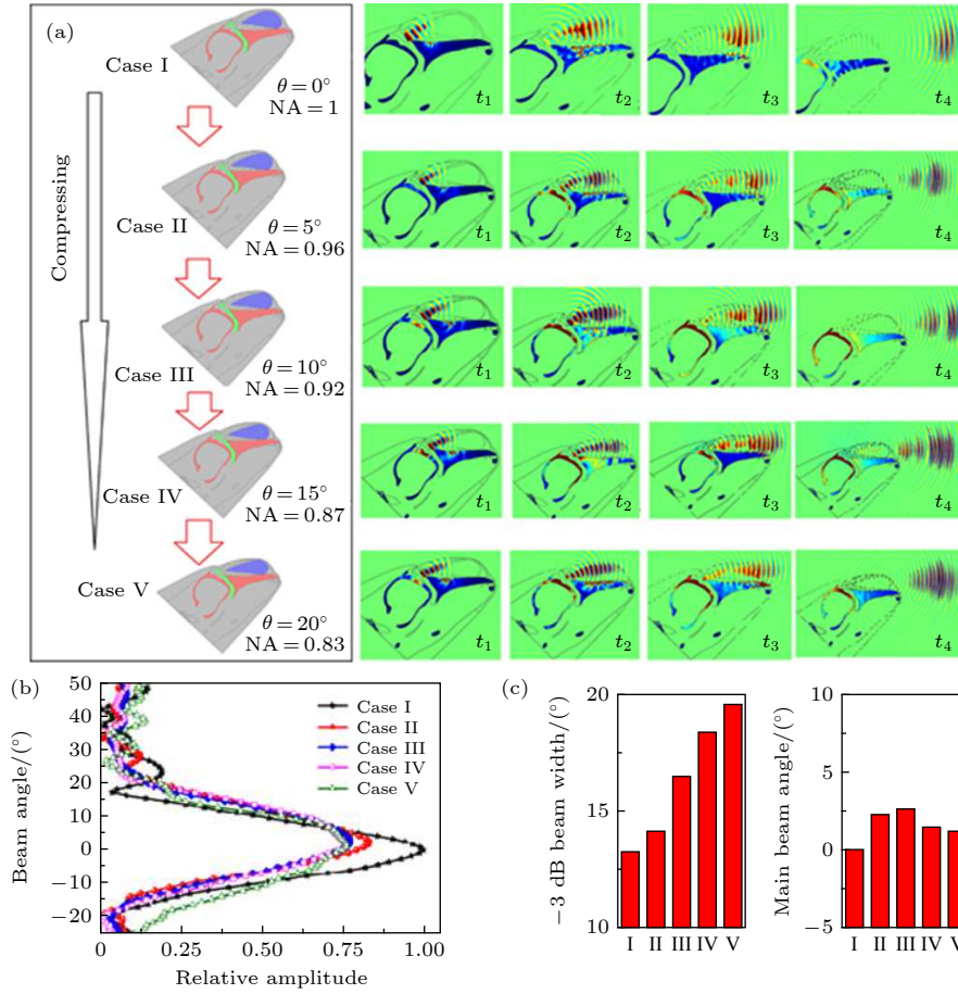
图 13 (a) 头部压缩对峰值频率为 125 kHz 的声脉冲传播形成的声场的影响, 其中 \theta 表示的是前庭囊的倾斜角, NA 代表的是相对于原始模型的归一化面积; (b) 五种模型相应的波束分布特性; (c) 五种模型形成的声波波束的 -3 dB 带宽与主瓣角分布 [34]
