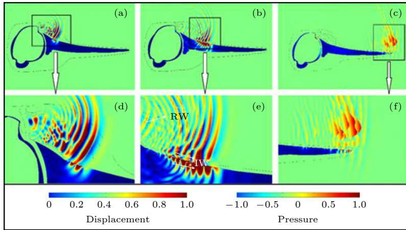
图 9 (a) 声波在白黵豚垂直截面第一传播时刻的声场分布; (b) 声波在白黵豚垂直截面第二传播时刻的声场分布, 其中 RW 与 IW 分别表示传播过程中的反射波与表面波; (c) 声波在白黵豚垂直截面第三传播时刻的声场分布; (d) 第一传播时刻声场分布放大; (e) 第二传播时刻声场分布放大; (f) 第三传播时刻声场分布放大 [74]
